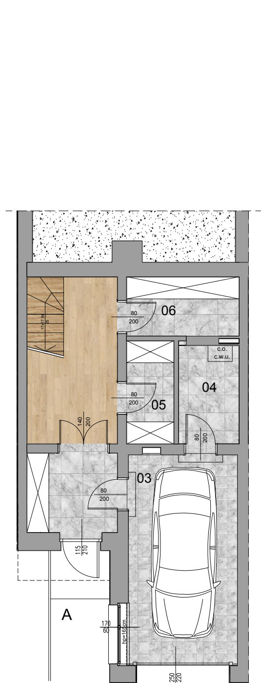
RZUT PARTERU
