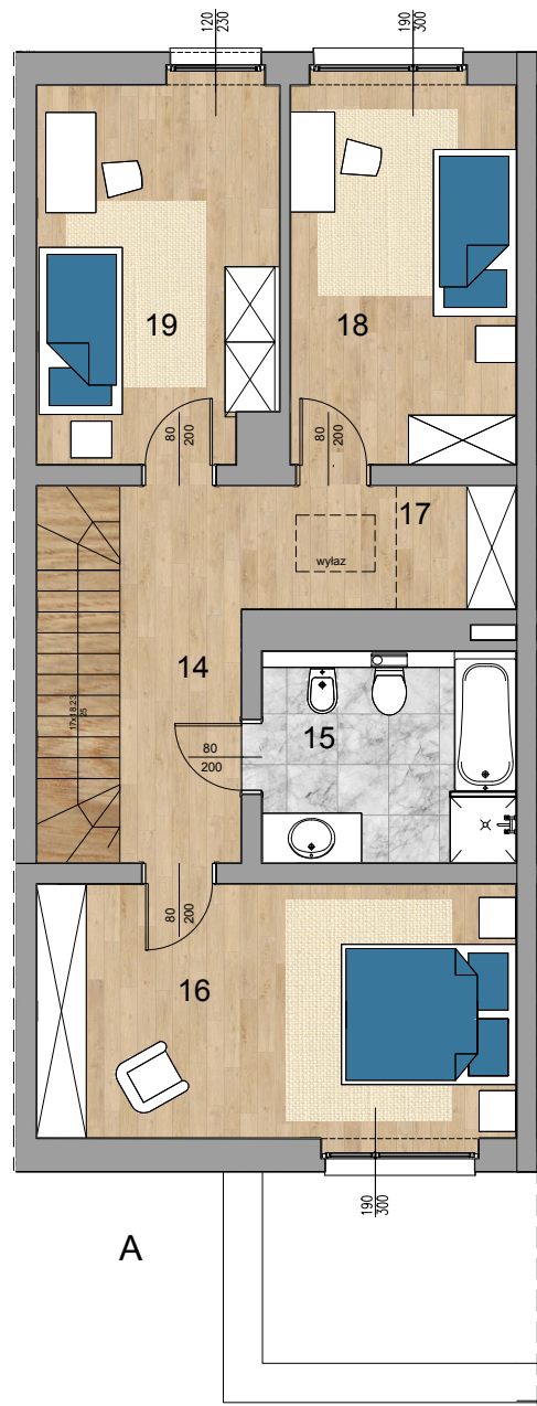
RZUT 2 PIETRA
