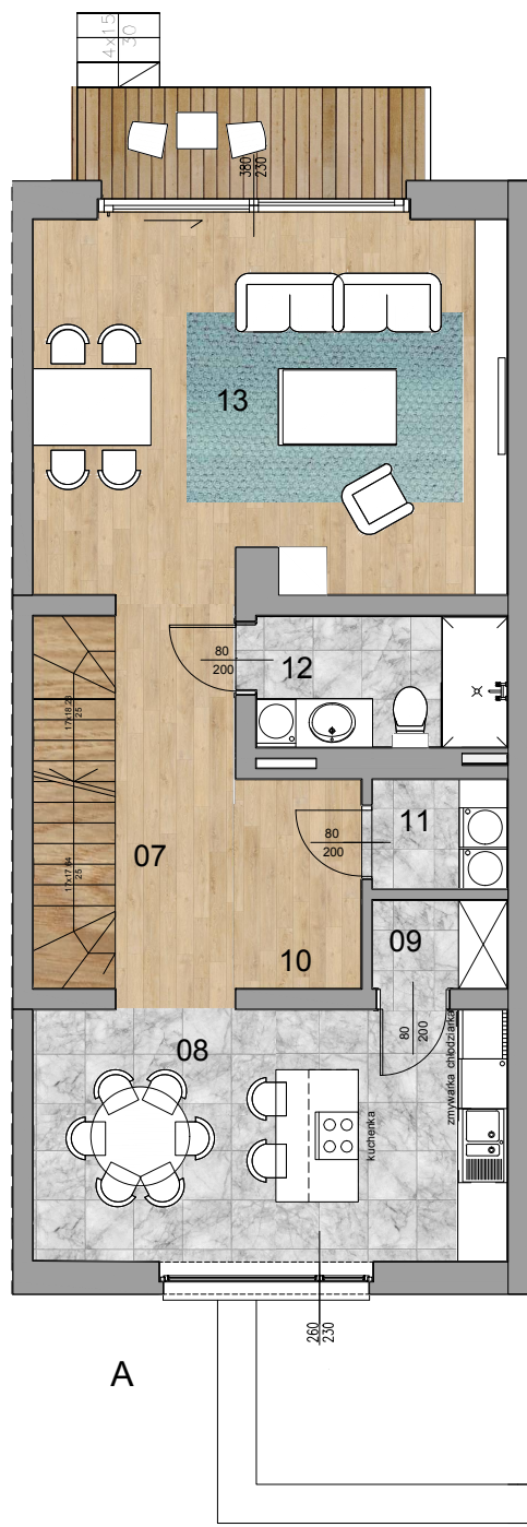
RZUT 1 PIETRA
