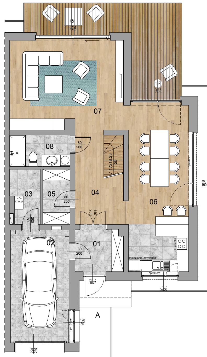
RZUT PARTERU
