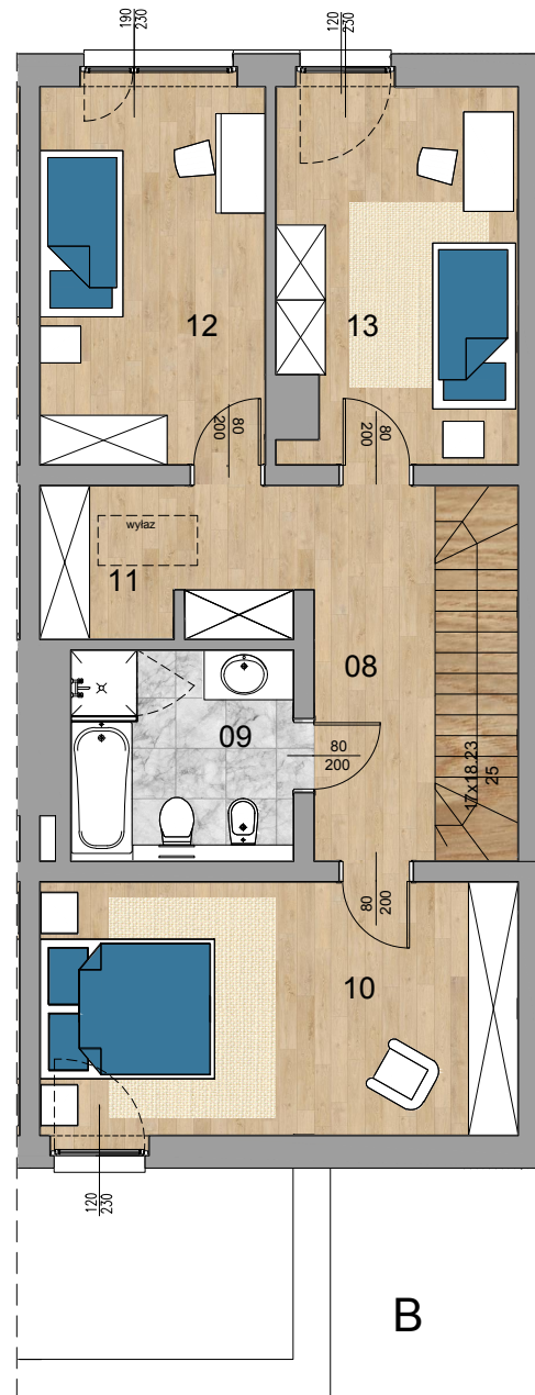
RZUT 1 PIETRA
