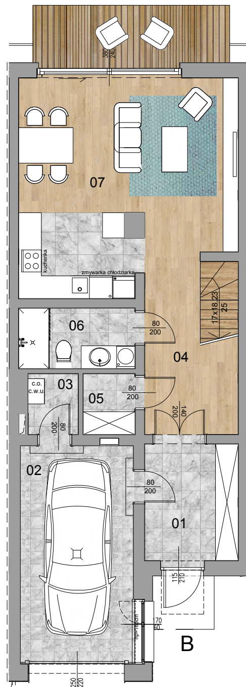
RZUT PARTERU
