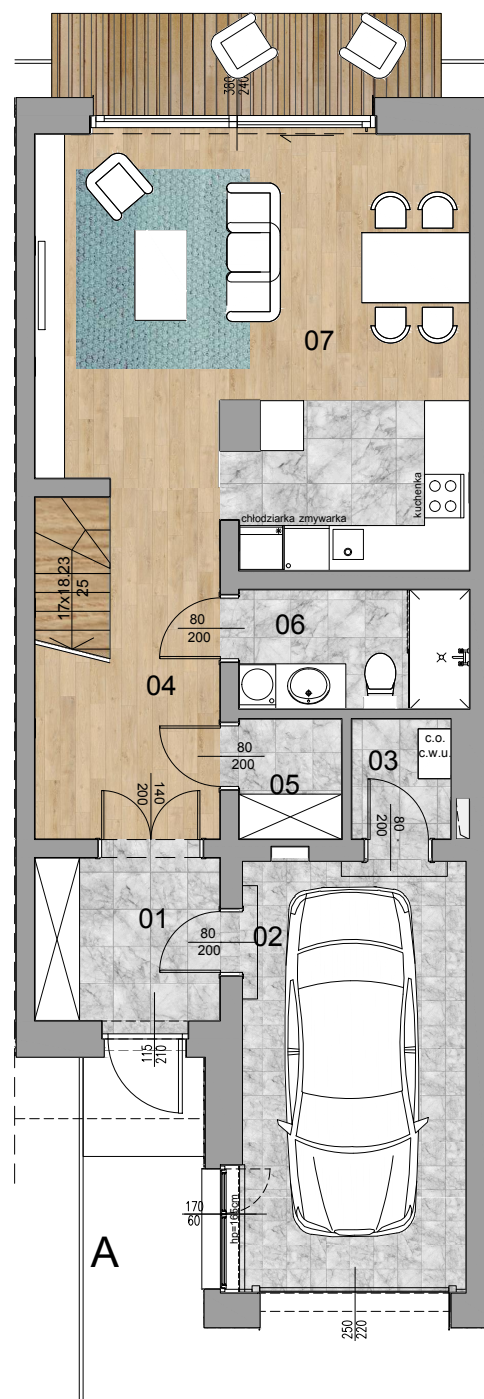
RZUT PARTERU
