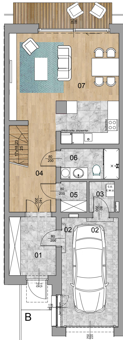
RZUT PARTERU
